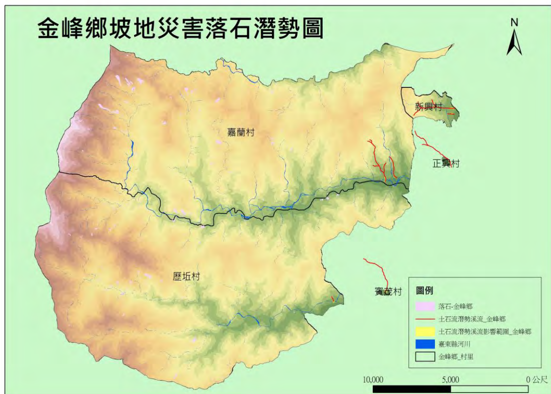
圖 1-8 金峰鄉坡地災害落石潛勢
