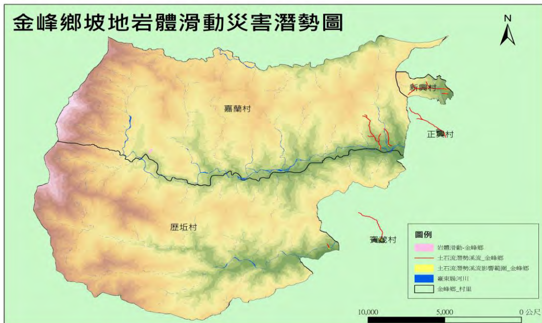
圖 1-10 金峰鄉坡地岩體滑動災害潛勢
